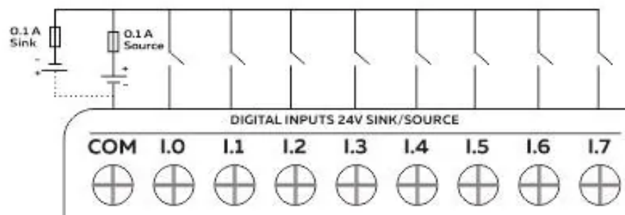
Cableado de la entrada digital NORVI-CEMA-M2
