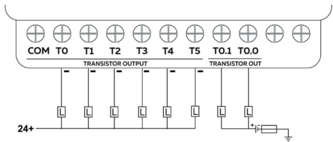
Cableado de salida del transistor NORVI-CEMA-M2
