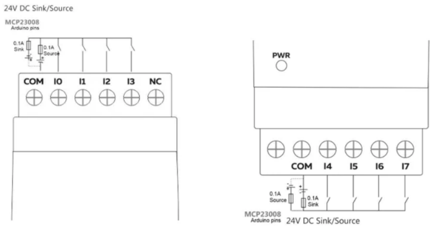
Cableado de la entrada digital EX-I8
